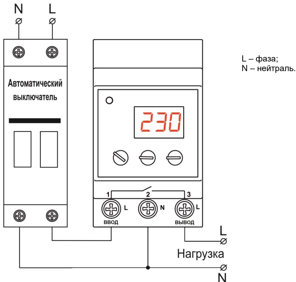
Рисунок 2 – Схема подключения РН-104(106)
