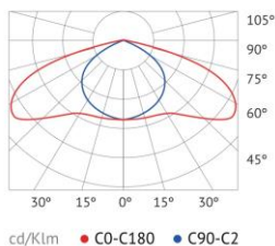
Кривая силы света
