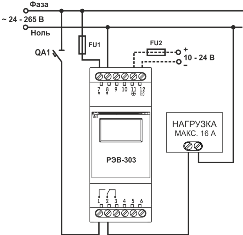
Рисунок 5.1 – Схема подключения РЭВ-303
