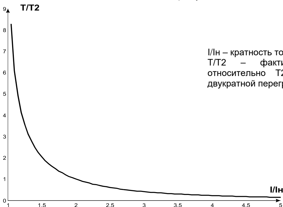
Рисунок 3.4 – Токо-временная характеристика
