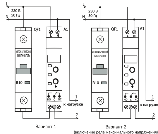
Вариант 2 (включение реле максимального напряжения)
