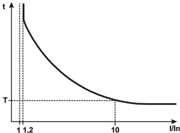
Рисунок 5 – Принцип работы защиты с зависимой выдержкой времени
