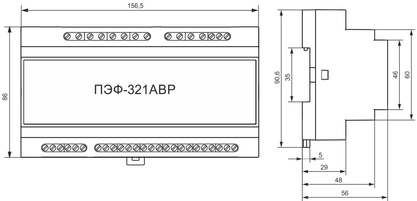
Рисунок 1 – Габаритные размеры ПЭФ-321ABP
