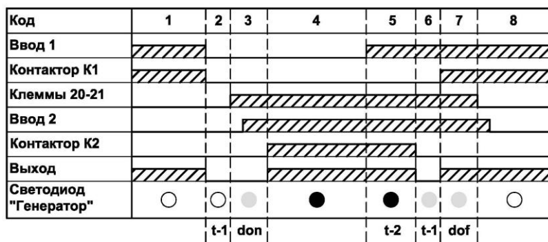
Рисунок 6 – Эпюры работы с генератором на вводе 2
